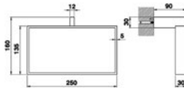
QU 090220 Porta Salviette Towel Ring Porte-Serviette
