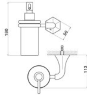
CE 090620 Dispenser Dispenser Diffuseur
