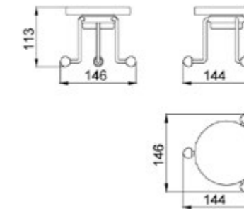
AR 090490 Porta Sapone Soap Holder Porte-Savon
