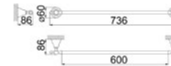
AR 090102 Porta Salviette Towel Rail Porte-Serviette
