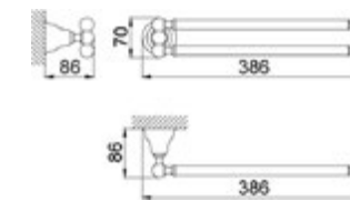
AR 090210 Porta Salviette Towel Rail Porte-Serviette
