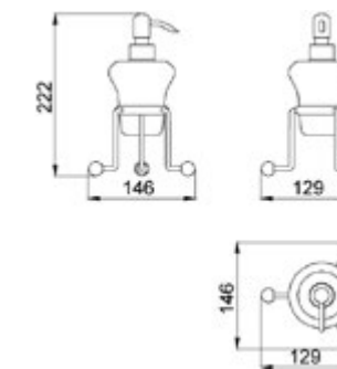
AR 090630 Dispenser Sapone Soap Dispenser Diffuseur de Savon
