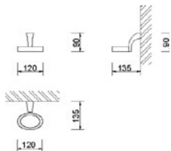
AE 090600 Porta Sapone Soap Holder Porte-Savon
