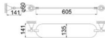
AR 090430 Mensola Shelf Console
