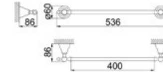
AR 090100 Porta Salviette Towel Rail Porte-Serviette
