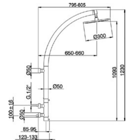
LN C91010 Colonna Doccia Termostatica Thermo Shower Column Colonne de Douche Thermo
