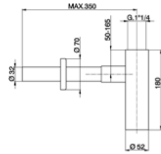
ZA 004070 Sifone Siphon Siphon
