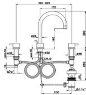
LN 001060 Batteria Lavabo Basin Set Lavabo 3 Trous
