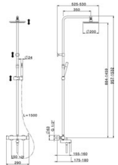
LN 004160 CombiVasca Monocomando CombiBath Mixer CombiBain Mitigeur
