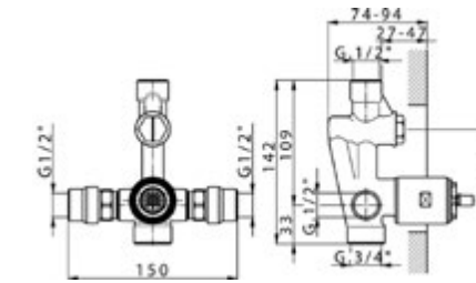
ZA 005211 Parte Incasso Monocomando 2 Uscite con Silenziatori 2-Outlet Mixer Concealed Part with Noise Reducers Partie Encastrée Mitigeur 2 Sorties avec Silencieux
