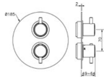
LN 018200 Parte Esterna Termostatico 3 Uscite 3-Outlet Thermo Exposed Part Partie Décor Thermo 3 Sorties
