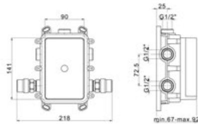
ZA 00B031 Parte Incasso ONE Box con Silenziatori ONE Box Concealed Part with Noise Reducers Partie Encastrée ONE Box avec Silencieux
