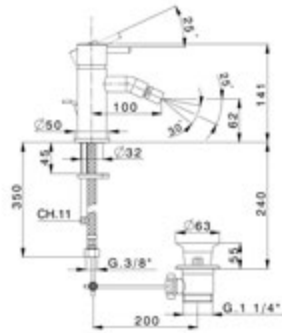
LN 000550 Monocomando Bidet Bidet Mixer Mitigeur Bidet
