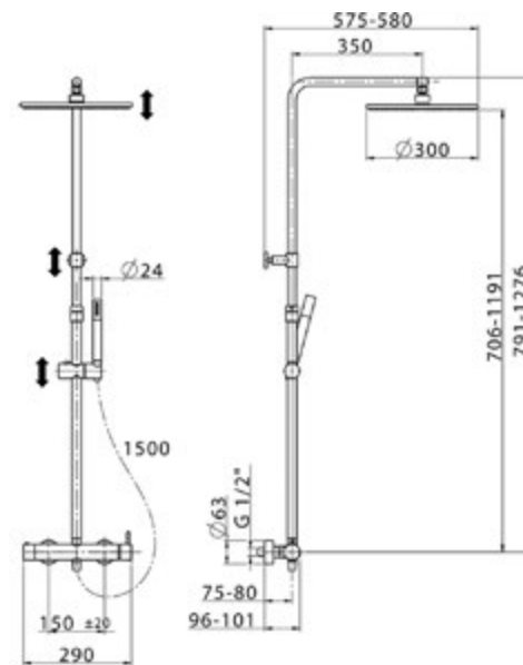
LN 004030 CombiDoccia Monocomando CombiShower Mixer CombiDouche Mitigeur
